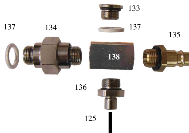
Anschlusssteil/Connecting part
